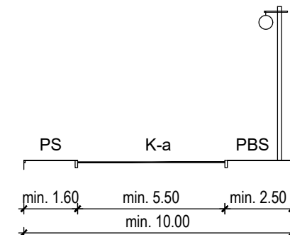
UK1 - presjek 1-1
